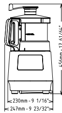
Alzado
